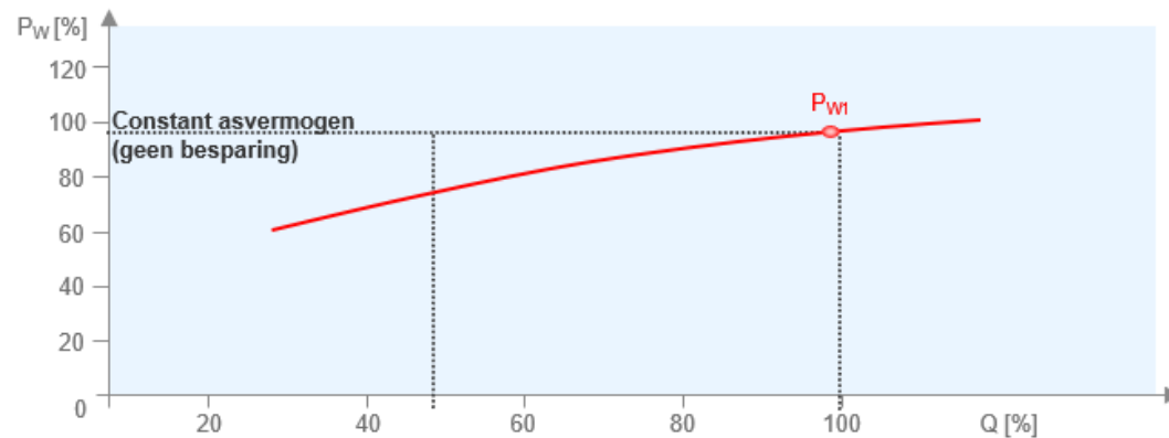
Grafiek: pomp- en vermogenscurve
