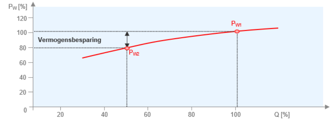
Grafiek: pomp- en vermogenscurve
